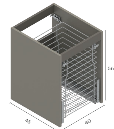
Bajo ropero
