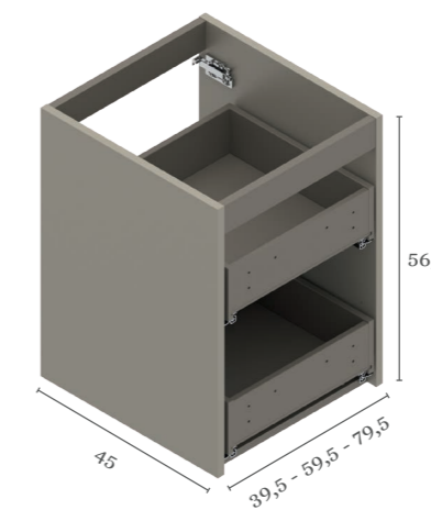
Bajo ropero
